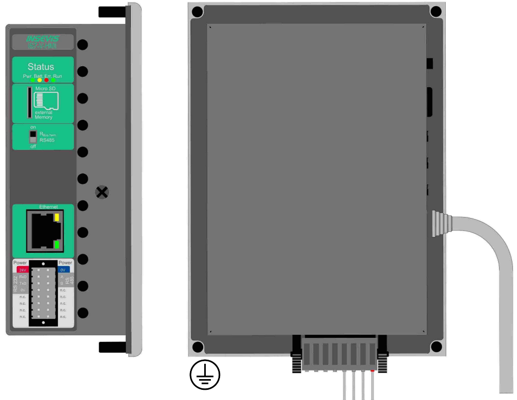
Bild oben: Ansichten des Touchpanels HMI350V im Vertikaleinbau von der Seite und von hinten
